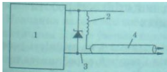
Рис. 87. Типовий захист обладнання з Живленням постійним током: 1 — джерело постійною струму; 2 — адіочастотна дросельна катушка; 3 — швидкодіючий варистор; 4 — екранований провід
