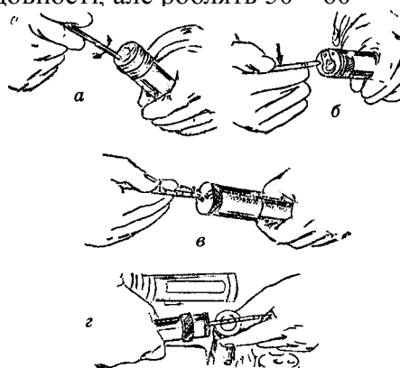
Рис. 20. Основні прийоми роботи з індикаторними трубками: a — надрізання кінців індикаторної трубок з допомогою ножа в насосі; б — обламування кінців індикаторних трубок; в — розбивання ампули індикаторних трубок; г — підсвічування ліхтарем вночі для визначення зміни забарвлення індикаторної трубки
