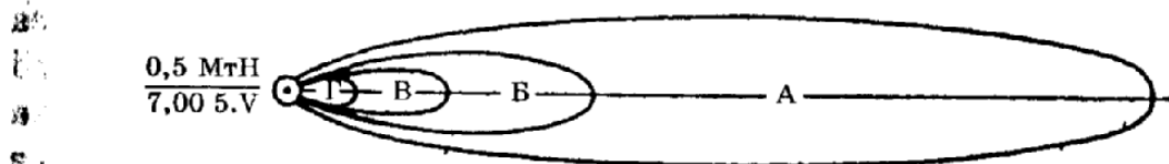
Рис. 23. Схема прогнозу зон радіоактивного забруднення ядерного вибуху
