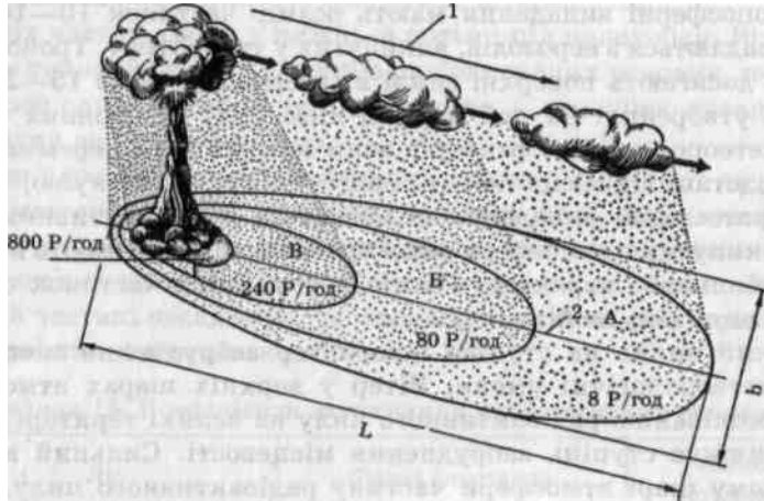
Рис. 7. Слід радіоактивної хмари наземного ядерного вибуху з рівнями радіації через 1 год після вибуху: 1 — напрямок середнього вітру; 2 — вісь сліду; А — зона помірного забруднення; Б — зона сильного забруднення; В — зона небезпечного забруднення; Г — зона надзвичайно небезпечного забруднення; L — довжина сліду; b — ширина сліду
