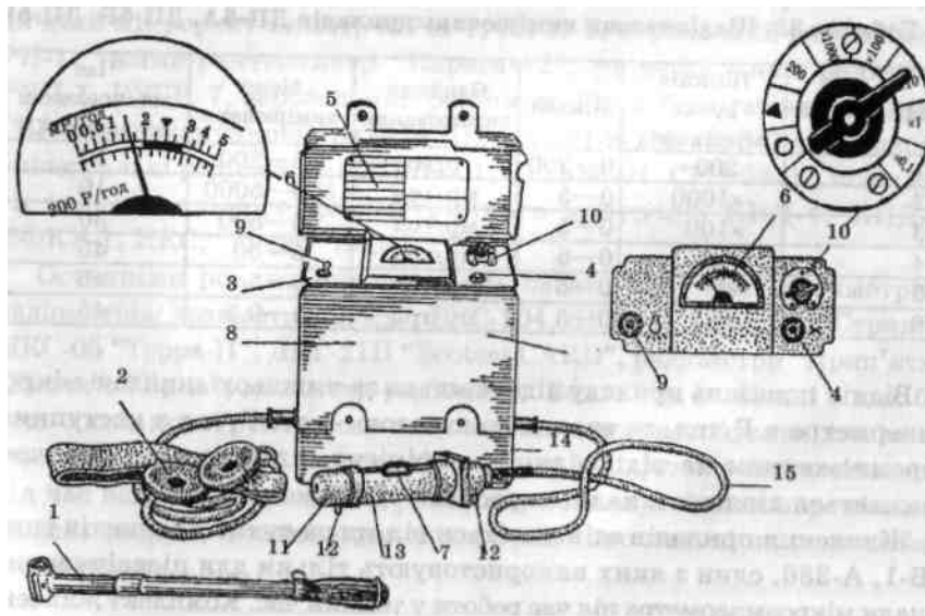
Рис. 11. Прилад ДП-5В:
