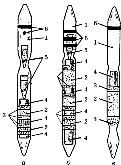
Рис. 19. Індикаторні трубки: а — з червоною крапкою і кільцем — для визначення зарину, зоману і Ві-Ікс; б — з трьома зеленими кільцями — для визначення синильної кислоти, хлорціану і фосфогену; в — з одним жовтим кільцем для визначення іприту; 1 — корпус трубки; 2 — наповнювач; 3 — ватні тампони; 4 — обтічник; 5 — ампули; 6 — маркіровочні кільця
