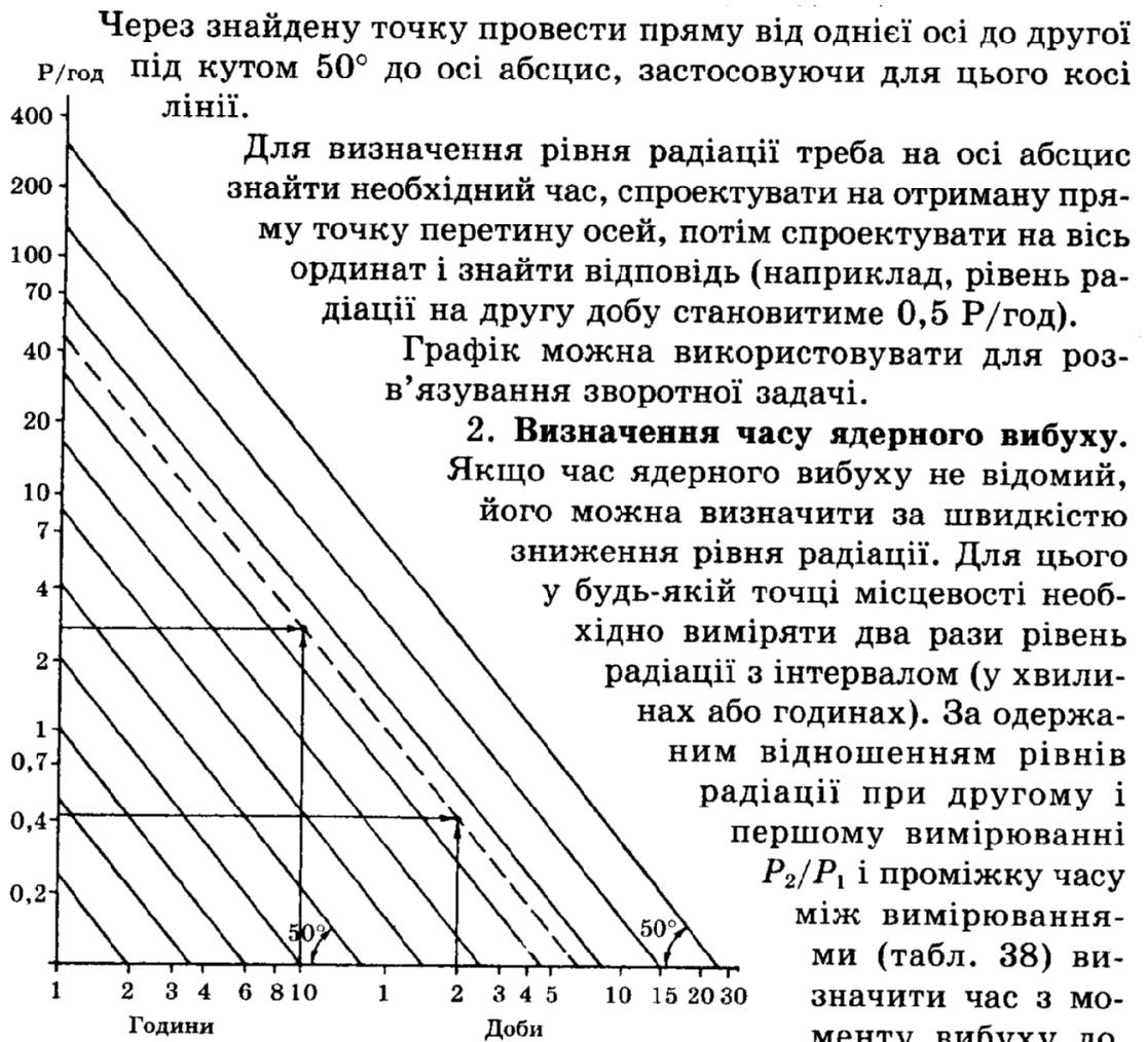
Рис. 24. Графік для визначення рівня радіації на будь-який час після вибуху
