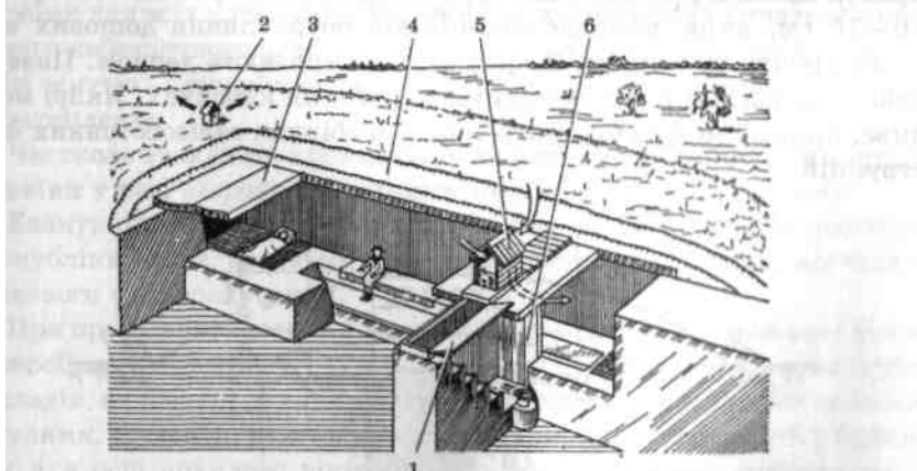
Рис. 37. Протирадіаційне укриття з перекриттям із залізобетонних плит: 1 — вхід; 2 — витяжна шахта; 3 — перекриття; 4 — обсіпка ґрунтом; 5 — припливна шахта; 6 — завіса при вході
