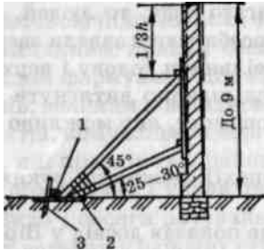
Рис. 93. Укріплення стіни по двійним підкосом: 1 — лежень; 2 — опорний брус 3 — паля
