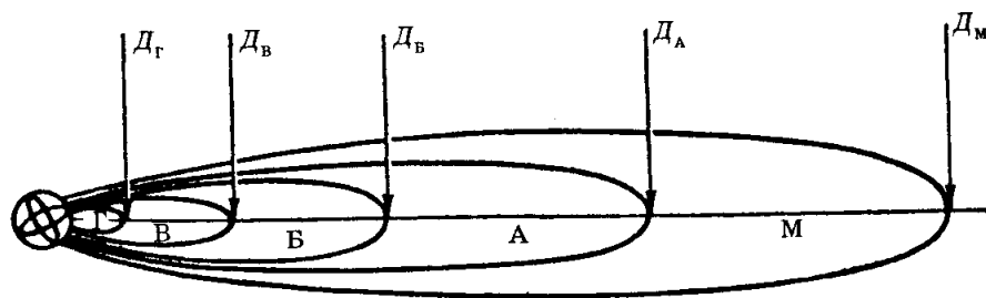
Рис. 28. Схема нанесення значення потужності доз випромінювання на зовнішніх межах зон радіоактивного забруднення після аварії на АЕС
