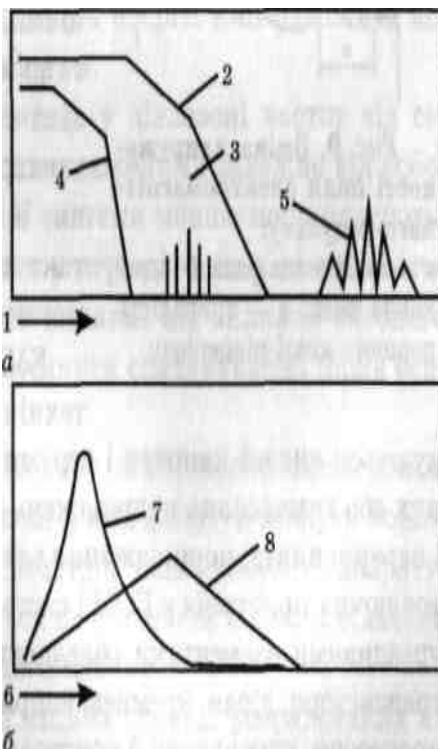
Рис. 8. Характеристика ЕМІ: а — порівняння частотних характеристик: 1 — частота; 2 — ЕМІ; 3 — засоби зв'язку; 4 — розряд атмосферної блискавки; 5 — радіолокатори; б — порівняння форм хвиль: 6 — час; 7 — ЕМІ; 8 — розряд атмосферної блискавки
