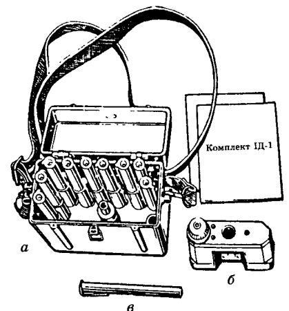
Рис. 14. Комплект індивідуальних дозиметрів ІД-1: a — загальний вигляд комплекту; б — зарядний пристрій ЗД-6; в — дозиметр
