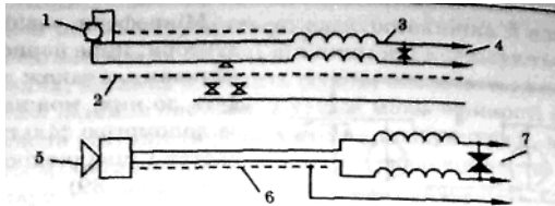
Рис. 89. Схема захисту ліній мікрофонів і репродукторів: 1 — мікрофон; 2 — екранована пара проводів; 3 — швидкодіючий варистор; 4 — до радіоустановки; 5 — зовнішній репродуктор; 6 — екранована пара проводів; 7 — до радіоустановки
