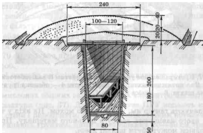
Рис. 38. Перекрита щілина
