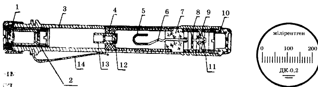
Рис. 17. Будова дозиметра ДК-0,2:
