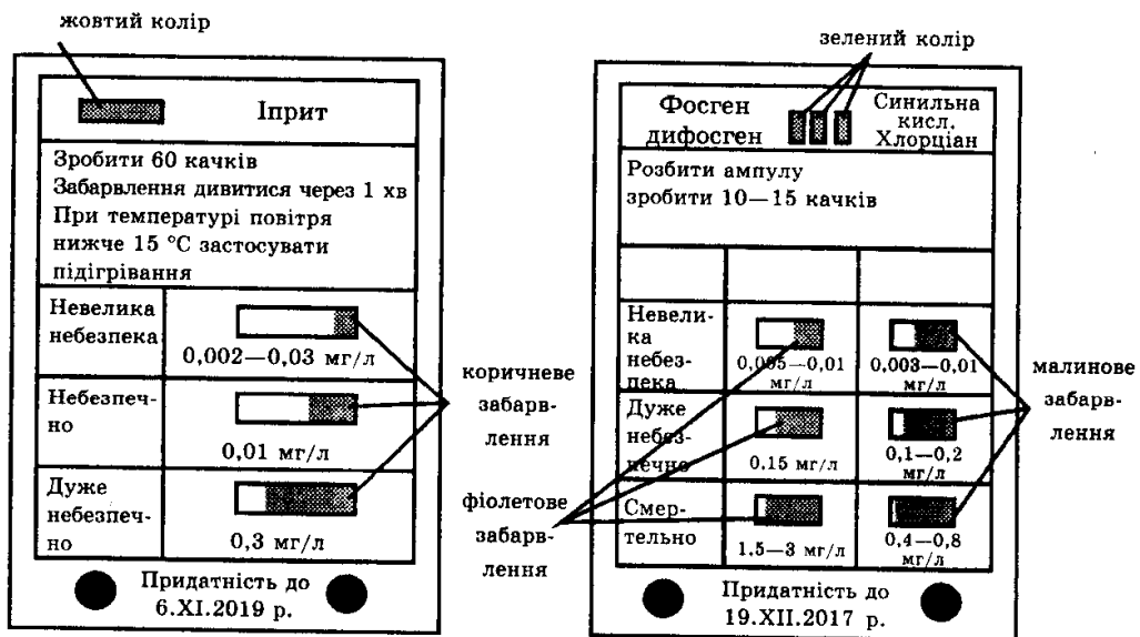
Рис. 21. Еталони забарвлення від ОР наповнювачів індикаторних трубок
