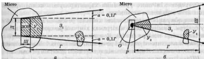
Рис. 10. Схема зони хімічного зараження і осередку хімічного ураження:
