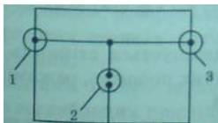
Рис. 88. Захист антени: 1 — антена; 2 — приймальний пере датчик, газорозрядна лампа
