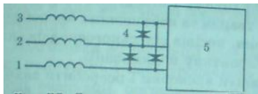
Ліс. 80. Захист вихідних силових кабельних ліній: 1 — фазний провід; 2 — централь; 3 — земля; 4 — швидкодіючий варистор; 5 — обладнання, що захищ.чстьс;І
