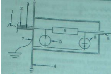
Рис. 86. Захист вихідних силових кабельних ліній: 1 — фазний провід; 2 — централь; 3 — земля; 4 — швидкодіючий варистор; 5 — обладнання, що
