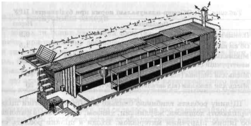
Рис. 36. Протирадіаційне укриття з тонких колод або жердин
