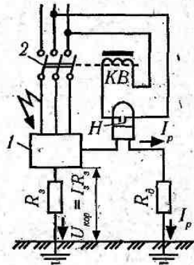
Рис. 3.28. Схема пристрою захисного вимкнення, який реагує на напругу корпусу відносно землі
