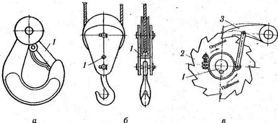
Рис. 3.5. Запобіжні пристрої вантажопідйомального обладнання:
