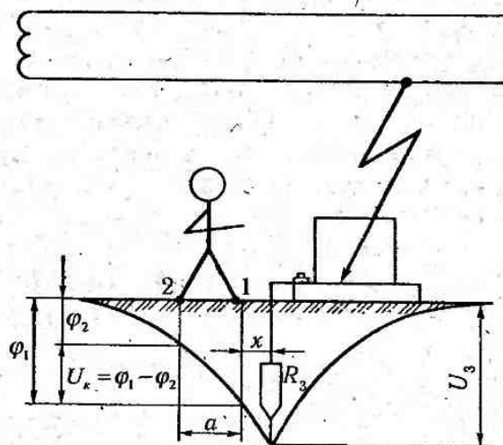
Рис. 3.18. Напруга кроку
