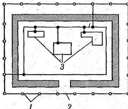
Рис. 3.26. Виносне (а) та контурне (б) заземлення: 1 — заземлювачі; 2 — заземлювальні провідники; 3 — устаткування
