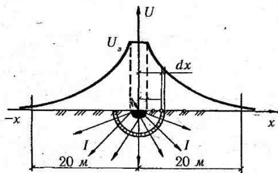
Рис. 3.16. Розтікання струму в ґрунті через напівсферичний заземлювач
