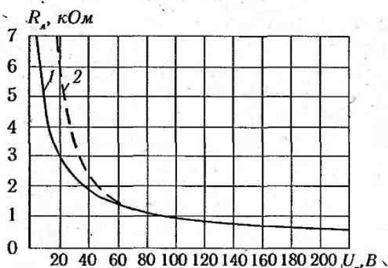
Рис. 3.9. Залежність опору тіла людини R_n від прикладеної напруги U_n : 1 — змінний струм 50 Гц; 2 — постійний струм
