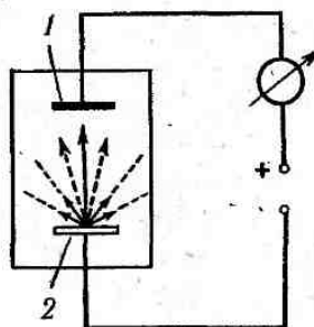
Рис. 4.30. Іонізаційна камера радіоізотопного сповіщувача диму:
