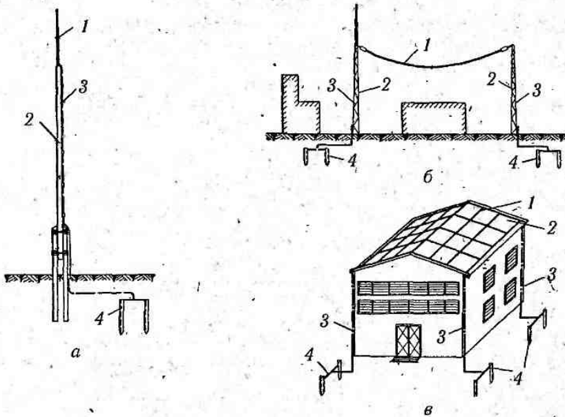
Рис. 3.35. Блискавковідводи:
