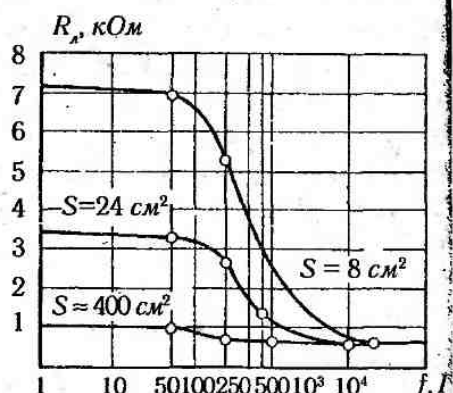
Рис. 3.10. Залежність опору тіла людини R_n на шляху струму «рука—рука» від частоти струму f та площі контакту S .
