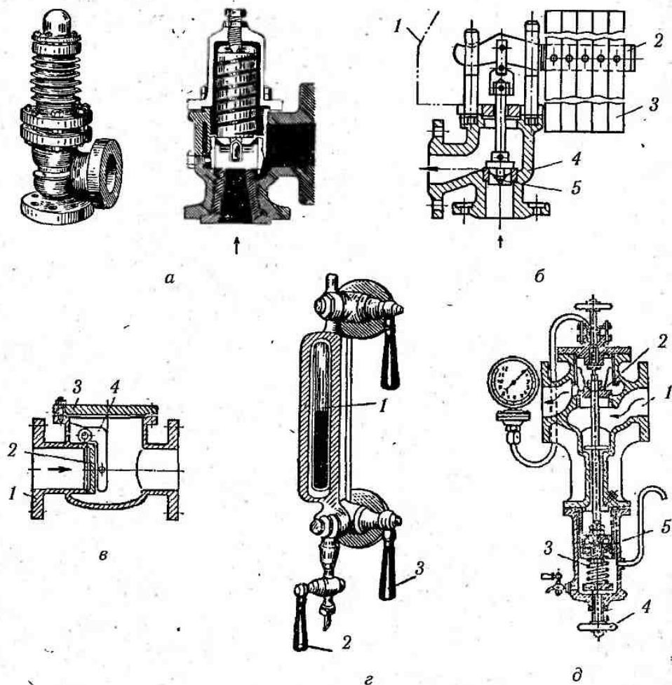
Рис. 3.1. Контрольно-вимірювальні прилади та запобіжні пристрої:
