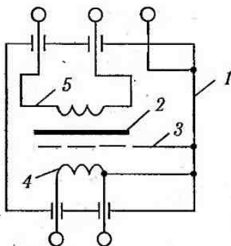
Рис. 3.21. Схема трансформатора малої напруги
