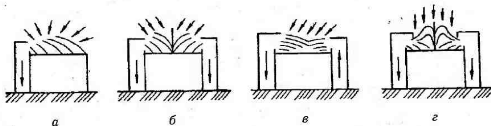
Рис. 2.13. Бортові відсмоктувачі: а — односторонній; б — двобортовий; в — з передувом; г — перевернутий
