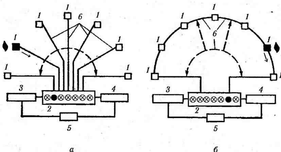
Рис. 4.27. Схеми променевого (а) та кільцевого (б) з'єднання в АУПС: 1 — сповіщувачі; 2 — приймально-контрольний прилад; 3 — блок живлення від електромережі; 4 — блок аварійного живлення; 5 — система перемикачів з одного живлення на інше; 6 — з'єднувальні проводи
