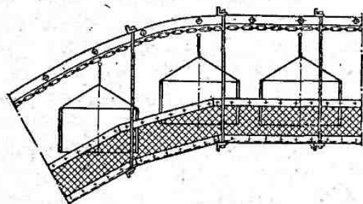
Рис. 3.6. Захисне огороження підвісного конвеєра
