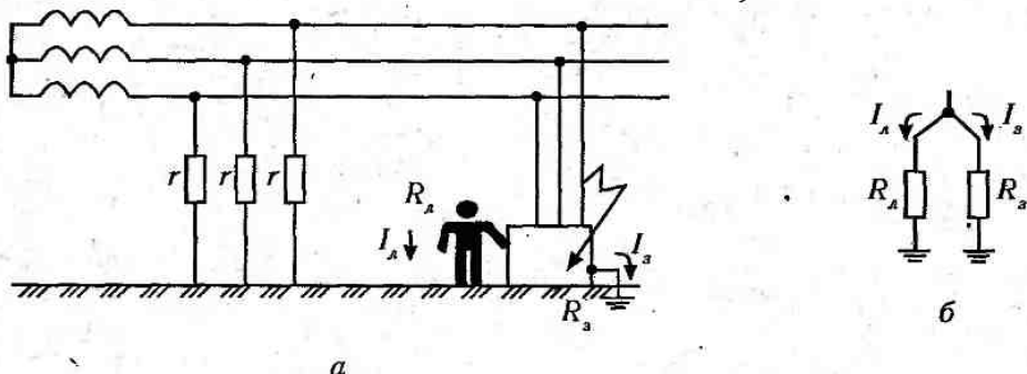
Рис. 3.24. Захисне заземлення:
