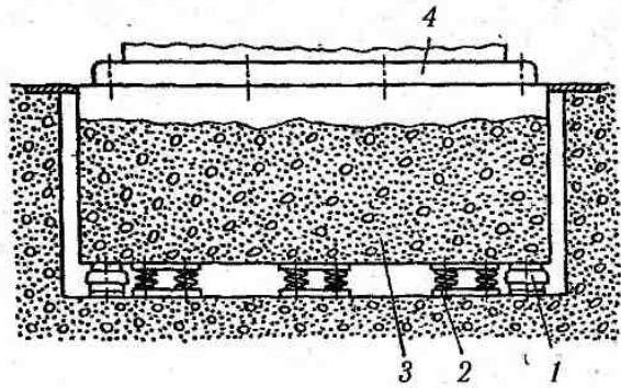
Рис. 2.28. Схема фундаменту під важкий металлооброблювальний верстат: 1 — амортизатори, 2 — пружини, 3 — фундаментна плита, 4 — станина верстату
