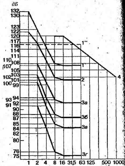
Рис. 2.25. Гігієнічні норми вібрації: 1—3 — загальна вібрація: 1' — вертикальна транспортна; 1'' — горизонтальна транспортна; 2 — транспортно-технологічна; 3а — технологічна у виробничих приміщеннях; 3б — у службових приміщеннях на суходолі; 3в — у виробничих приміщеннях, де немає джерела вібрації; 3г — у приміщеннях адміністративно-управлінських та для розумової праці; 4 — локальна вібрація.
