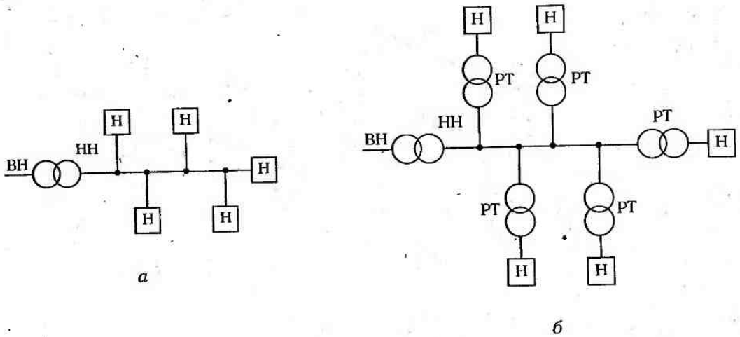
Рис. 3.23. Схема електричної мережі до (а) та після (б) поділу: Н — навантаження; РТ — роздільний трансформатор; ВН — мережа високої напруги; НН — мережа низької напруги
