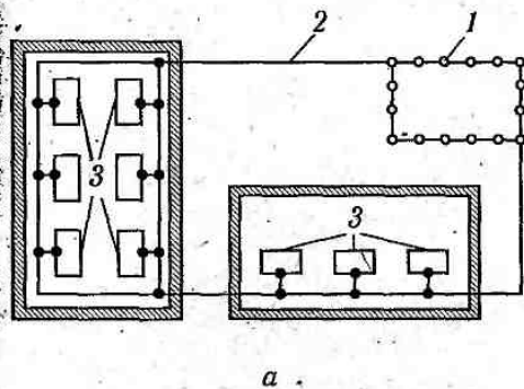
Рис. 3.26. Виносне (а) та контурне (б) заземлення: 1 — заземлювачі; 2 — заземлювальні провідники; 3 — устаткування
