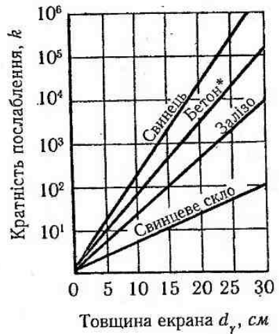
Рис. 2.39. Монограма для визначення товщини захисного екрана від гамма-випромінювання радія (* — для бетону d_\gamma множитьесь на 4)
