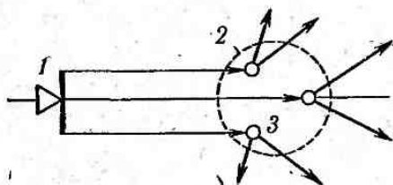
Рис. 4.29. Розсіювання світлового потоку частинками диму:
