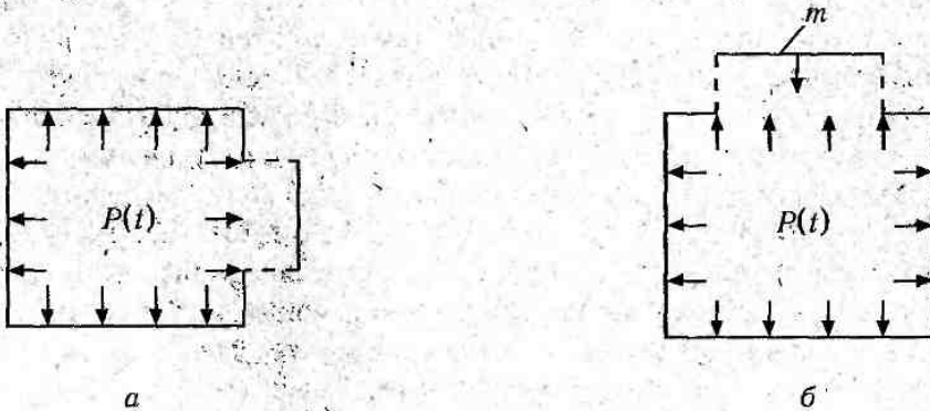
Рис. 4.16. Схеми дії настінних (а) та покрівельних (б) легкоскидних конструкцій
