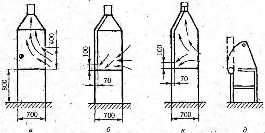
Рис. 2.11. Витяжні шафи:
