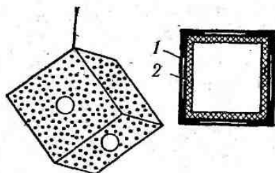
Рис. 2.38. Штучний звукопоглинач: 1 — перфорований корпус; 2 — звукопоглинальний матеріал
