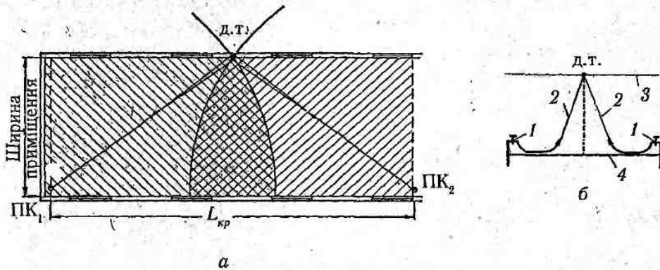
Рис. 4.26. Розміщення пожежних кранів та план зрошення приміщення, в якому вони встановлені: а — план зрошення приміщення двома пожежними кранами; б — схема зрошення диктуючої точки приміщення; 1 — пожежні крани; 2 — струмені води; 3 — стеля; 4 — підлога
