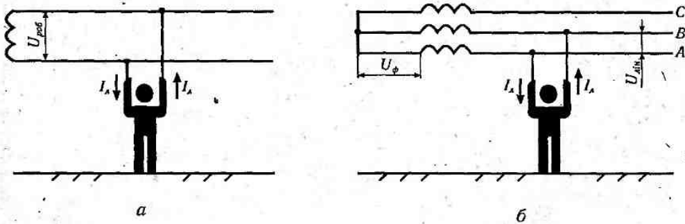
Рис. 3.13. Схема двофазного доторкання:
