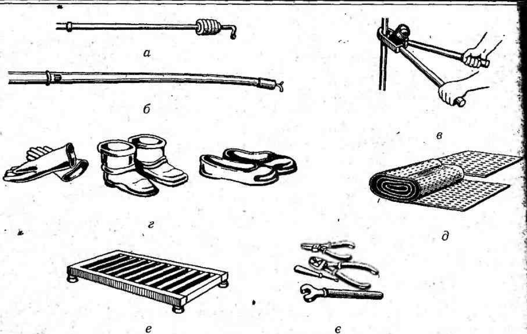
Рис. 3.29. Ізолювальні електрозахисні засоби:
