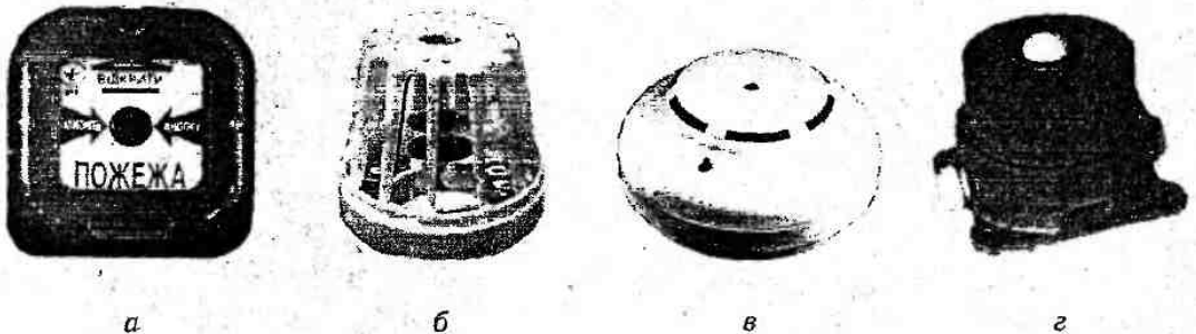
Рис. 4.28. Пожежні сповіщувачі: а — ручний ИП-П; б — тепловий ИП105; в — димовий ИПД-1; д — полум'я ИП
