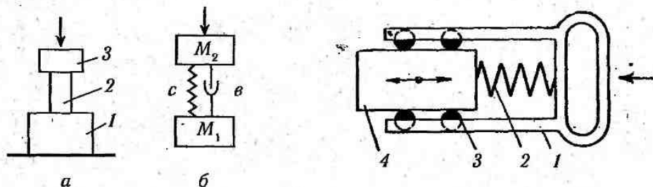
Рис. 2.30. Віброізований держак:
