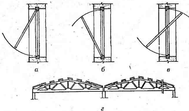
Рис. 4.17. Приклади легкоскидних конструкцій: верхньо — (а), нижньо — (б), та середньо підвісні (в) віконні рами; покриття покрівлі плитами ПНСЛ (д)
