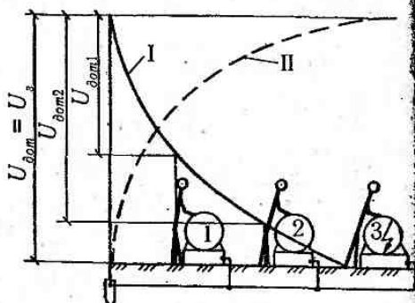
Рис. 3.17. Напряга доторкання до заземлених струмопровідних частин, що опинилися під напругою
