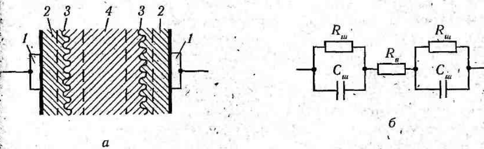
Рис. 3.8. Умовні схеми опору тіла людини:
