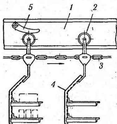
Рис. 3.7. Схема встановлення уловлювача на підвісному конвеєрі 1 — монорельс; 2 — ролики підвіски; 3 — привідний ланцюг; 4 — підвіски до виробів; 5 — гальмівний уловлювач
