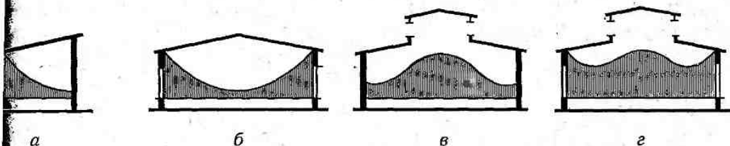
Рис. 2.17. Криві розділу освітленості в приміщеннях при різних видах природного освітлення:
