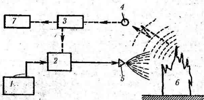
Рис. 4.18. Схема, що пояснює принцип дії автоматичної установки пожежогасіння:
