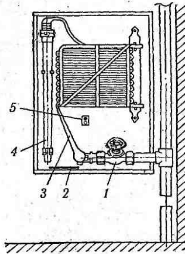
Рис. 4.25 Внутрішній пожежний кран 1 — вентиль; 2 — важіль для полегшення відкриття вентилля; 3 — пожежний рукав; 4 — ствол пожежний ручний; 5 — пульт дистанційного запуску насоса-підвищувача тиску
