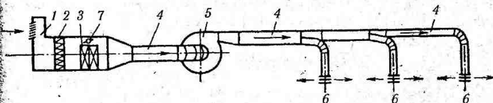
Рис. 2.7. Схема припливної вентиляції
