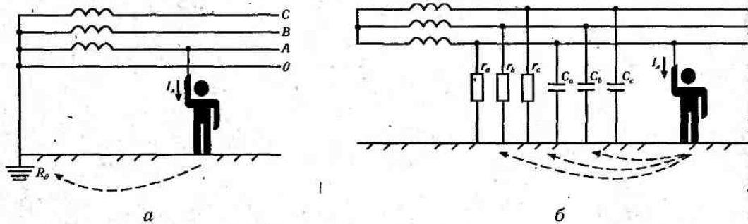
Рис. 3.14. Схема однофазного доторкання при нормальному режимі роботи: а — у трифазній мережі з глухозаземленою нейтраллю; б — у трифазній мережі з ізольованою нейтраллю
