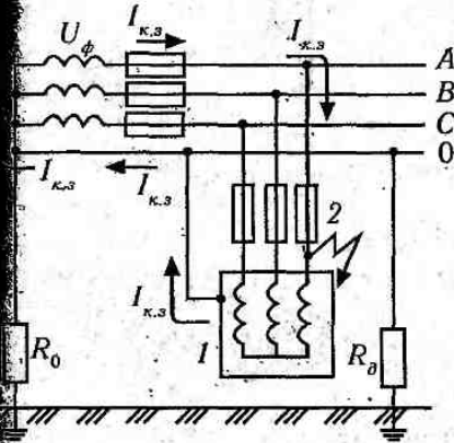
Рис. 3.27. Схема захисного занулення.
