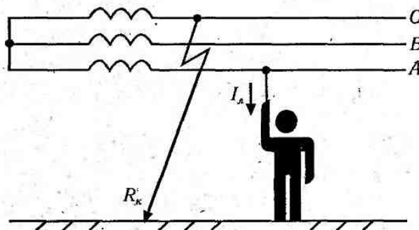
Рис. 3.15. Схема однофазного доторкання до справної фази несправної електромережі
