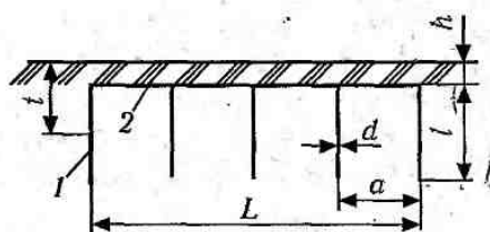
Рис. 3.25. Схема розташування заземлювачів: 1 — заземлювачі; 2 — заземлювальний провідник
