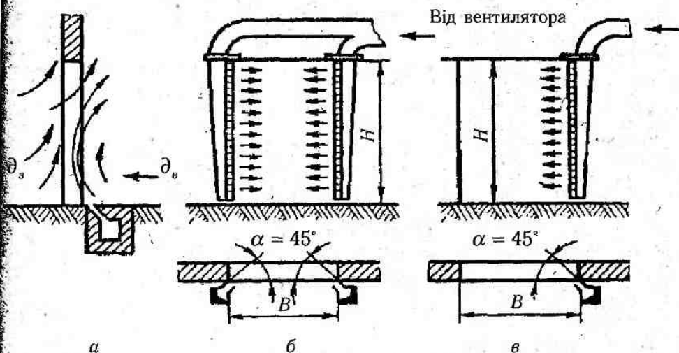
Рис. 2.9. Повітряно-теплові завіси:
