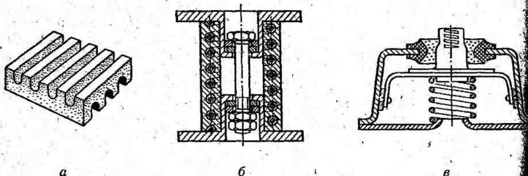
Рис. 2.31. Віброізоляційні амортизатори:
