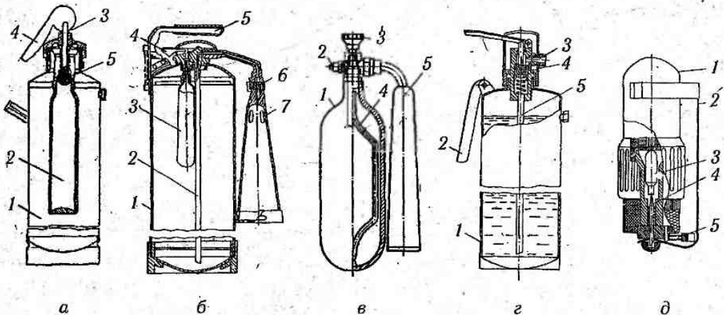
Рис. 4.22. Переносні вогнегасники:
