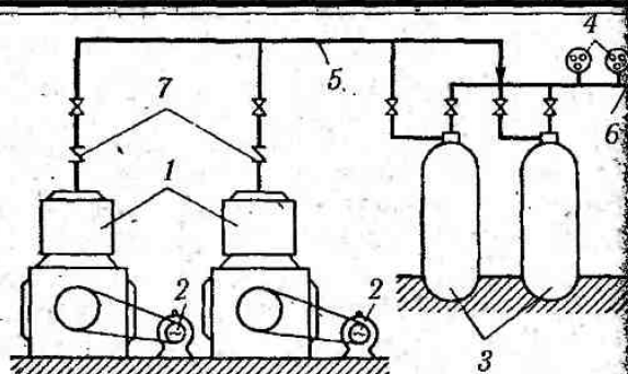
Рис. 3.3. Компресорна установка з автоматичним керуванням:
