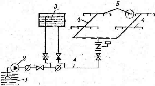
Рис. 4.19. Схема спринклерної установки
