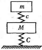
Рис. 2.27. Схема дії динамічного віброгасника
