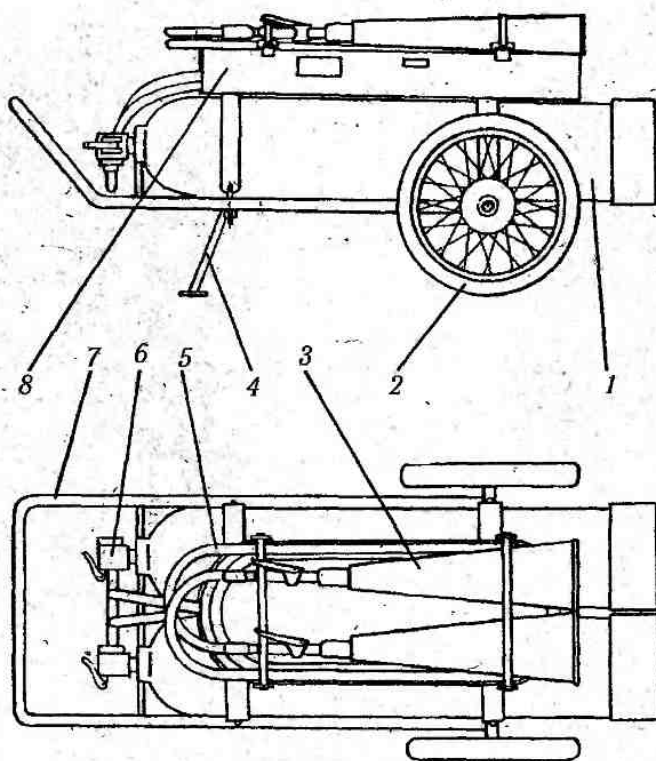
Рис. 4.21. Пересувний вогнегасник ДД-00.
